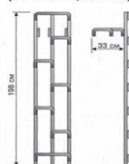
ВЛ Лестница Л-2 (Л-19) (водопроводная, водосточная)
